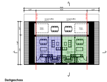
Dachgeschoss
