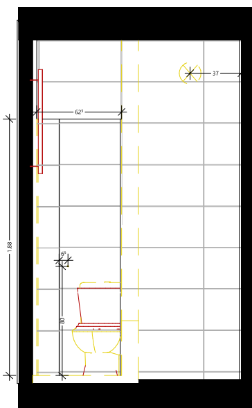
Ansicht 03
