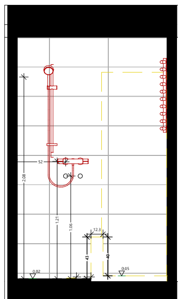
Ansicht 04
